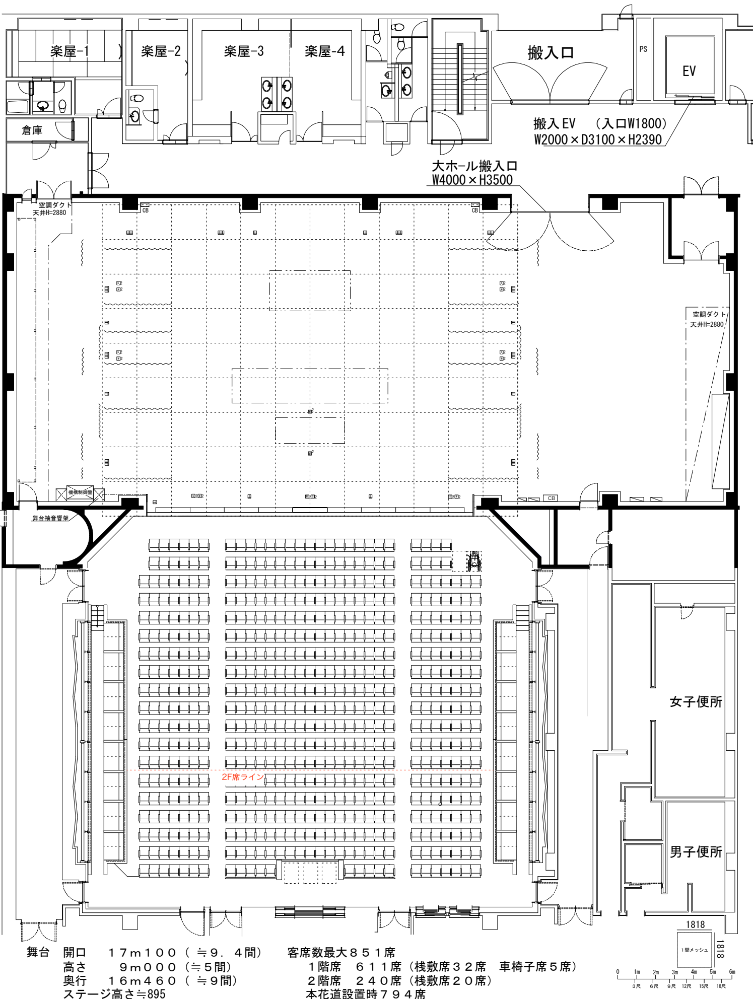
石川県こまつ芸術劇場 うらら 大ホール1階平面図
